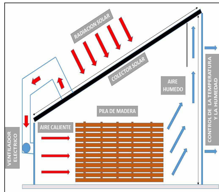
Diagrama operativo del horno solar construido en Tuapurie
